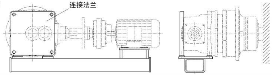
电机安装支架(附件代号—71)
