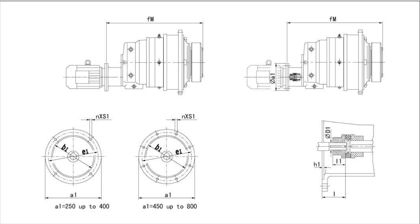
P2S. 带电机、输入法兰及联轴器尺寸
