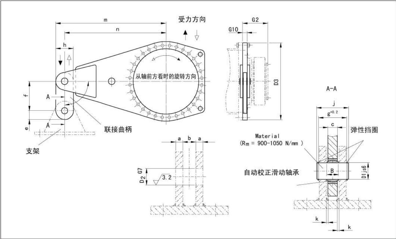
单向扭力臂 (附件代号—75)
