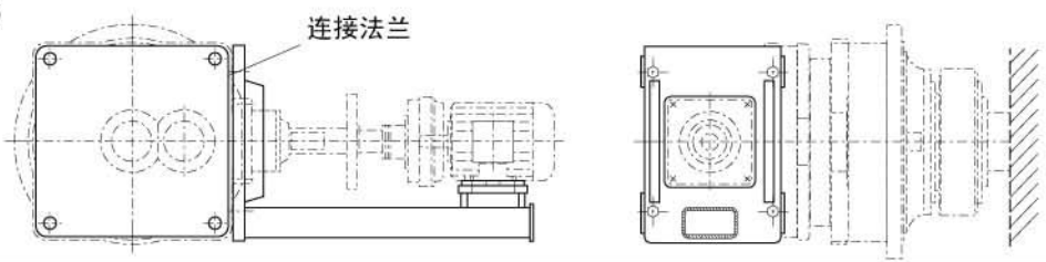
电机安装支架(附件代号—71)
