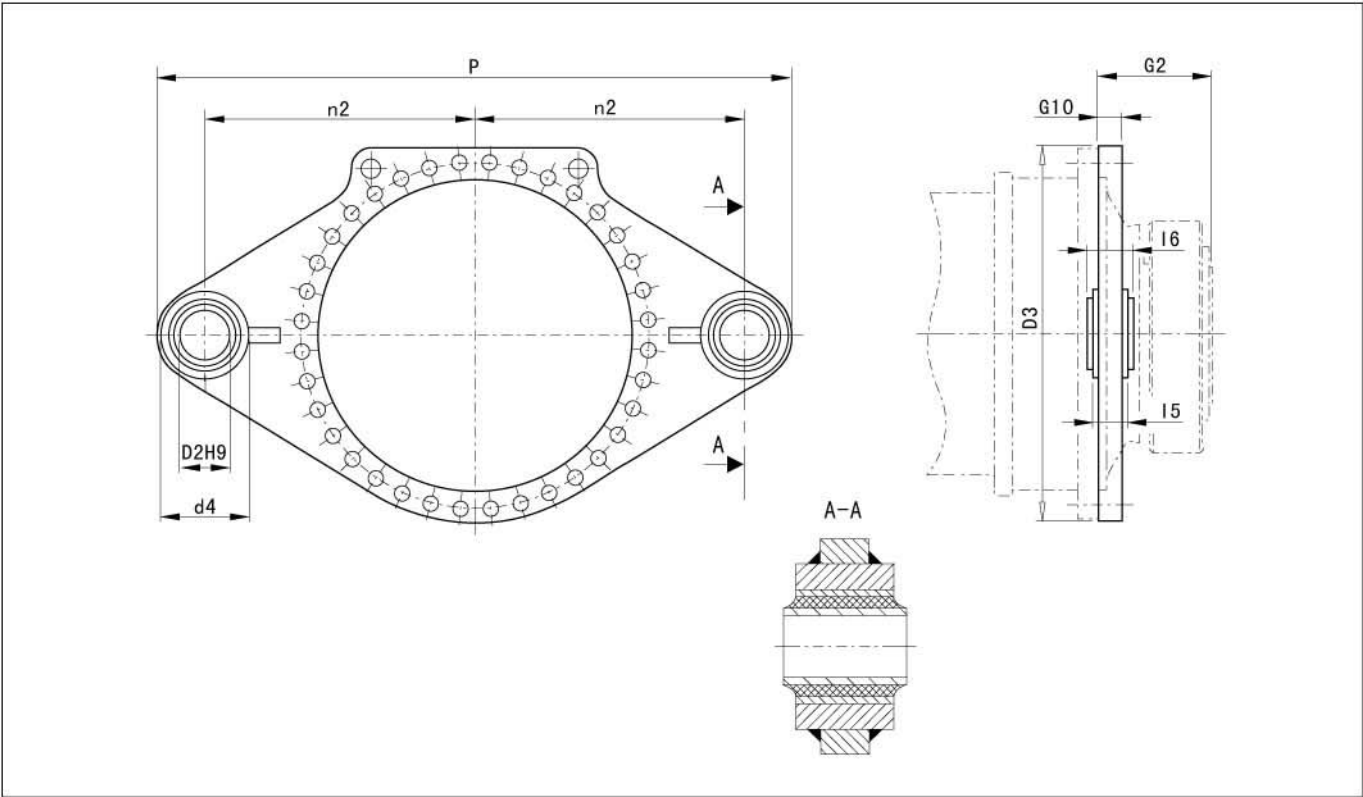
带橡胶衬套的双向扭力臂 (附件代号—76)
